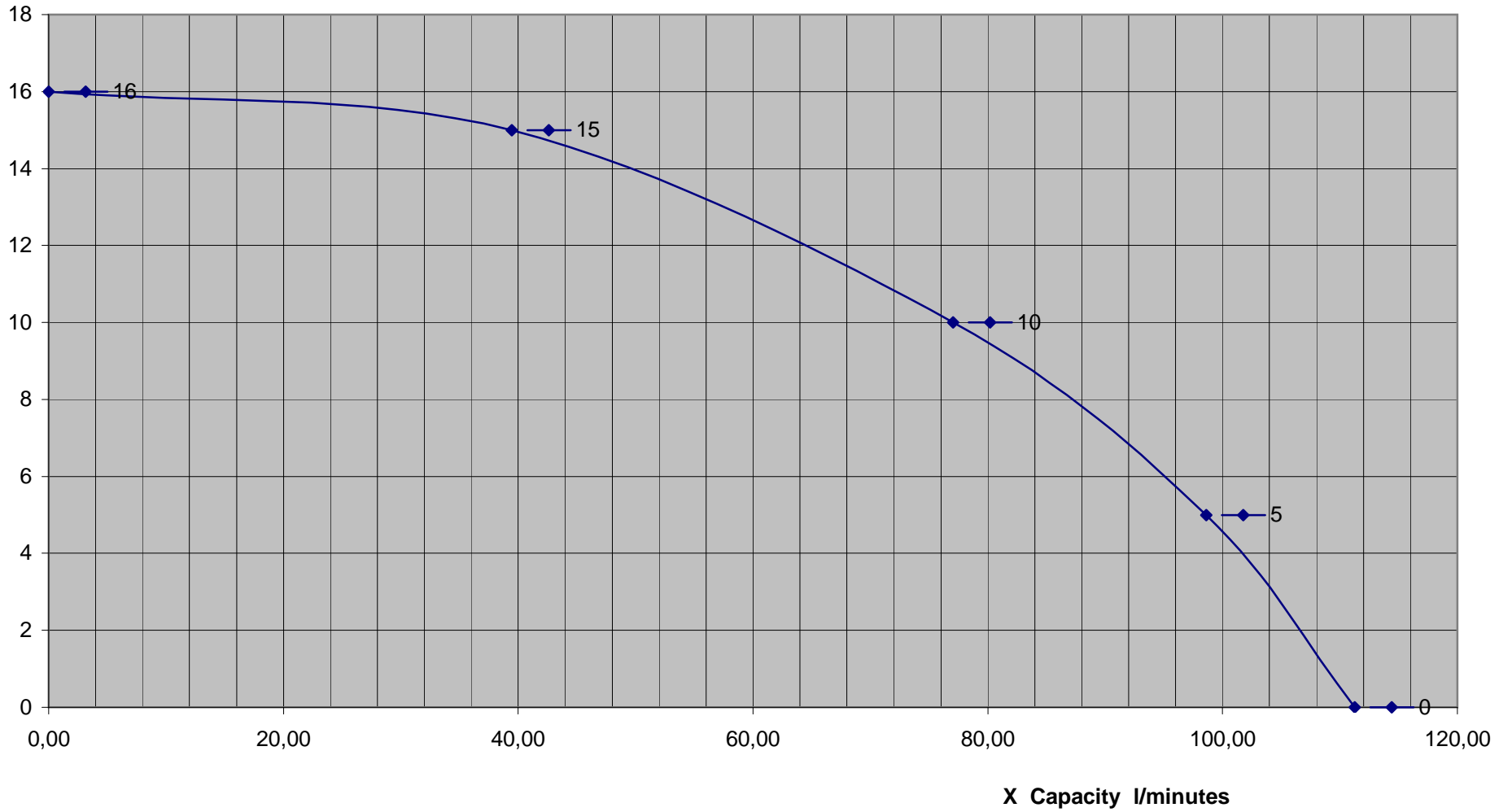
Pump Performance Data CESE3 HP 0,75 (Kw 0,55)
